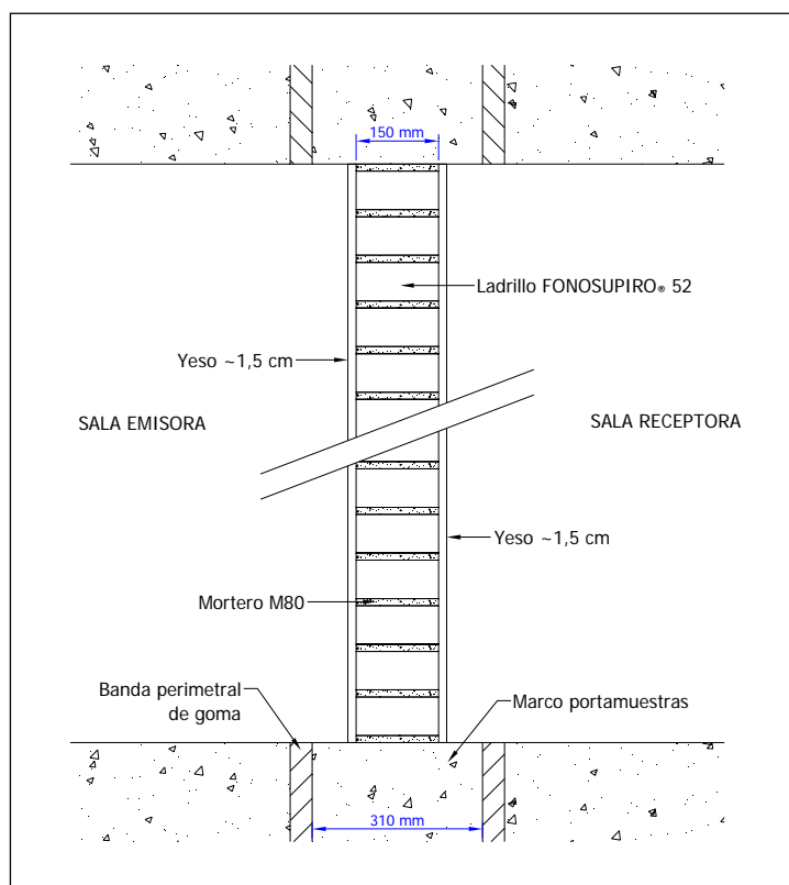
Figura 1 Sección de la pared construida en el laboratorio
